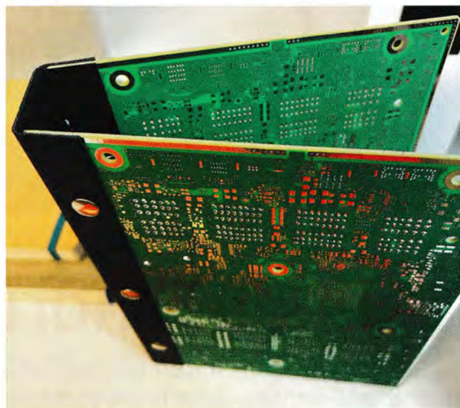
Mikroelektronik-Ringbuchordner: Seitens der Buchbinderei Bruder wurden die Platinen mit Einlage und Lederrücken verbunden, Platinen und Ringmechanik sind mit Nieten fixiert worden.
